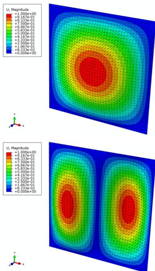
شکل ۵- مود شکل اول و دوم کمانش ورق فولادی
