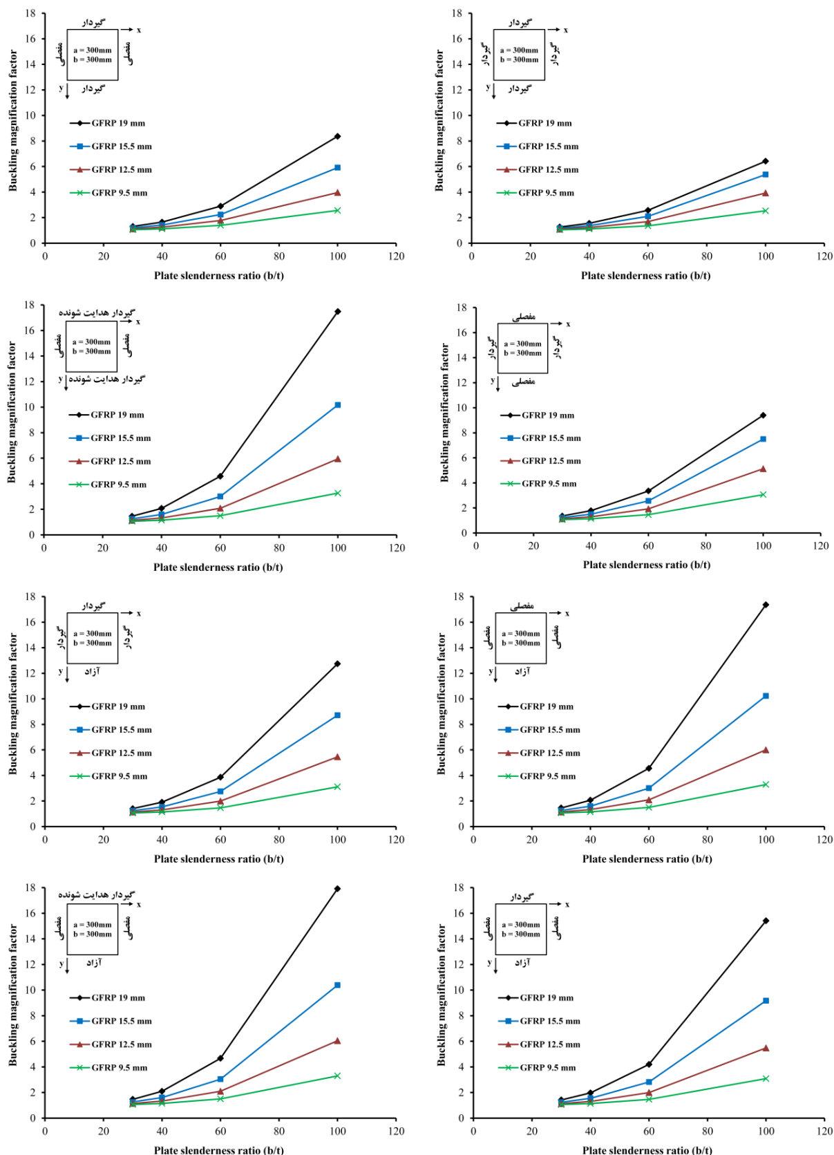
شکل ۱۳- تاثیر ورق GFRP بر افزایش ظرفیت کمانش ورق های نوع II
