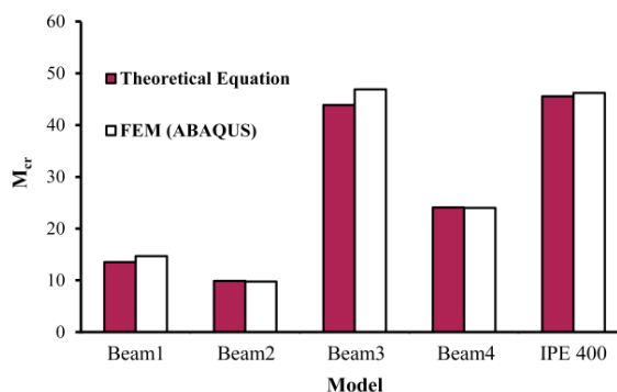
شکل ۸- مقایسه مقادیر لنگر کمانش پیچشی-جانبی بدست آمده از تحلیل در نرم‌افزار و رابطه‌های تئوری برای نمونه‌های مورد بررسی
