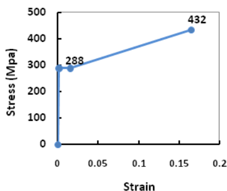
شکل (۱۸): مشخصات رفتار مکانیکی مصالح ستون، تیر و صفحه انتهایی
