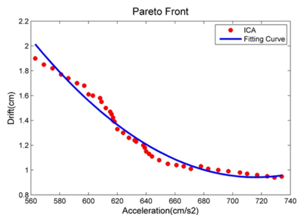
شکل ۸- جبهه بهینه پارتو برای حداکثر شتاب طبقات و حداکثر جابه‌جایی نسبی طبقات
