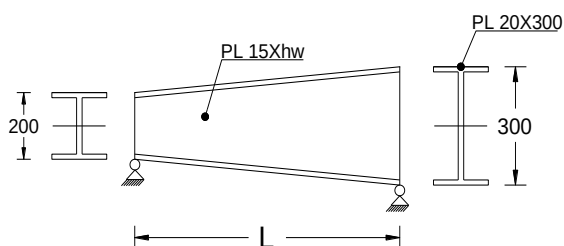
شکل ۸- عضو با مقطع متغیر پیوسته به ارتفاع جان ۳۰۰ میلی متر
