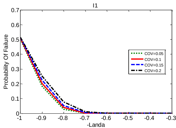
شکل ۱۰- محاسبه احتمال خرابی در سطوح مختلف نیرو کم‌انرژی و تأثیر پارامتر I_1 (برای شکل (۸))
