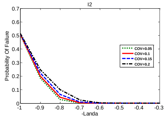
شکل ۱۶- احتمال خرابی در سطوح مختلف نیرو کمائی و تأثیر پارامتر I_2 (برای شکل (۱۳))
