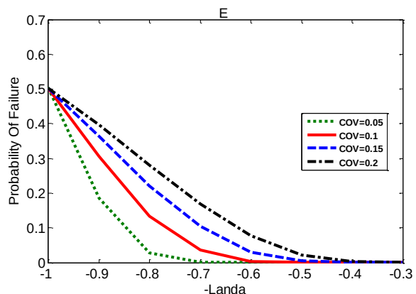
شکل ۱۷- احتمال خرابی در سطوح مختلف نیروی کمائی و تأثیر پارامتر L (برای شکل (۱۳))
