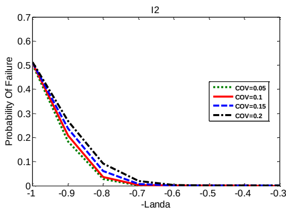
شکل ۱۱- احتمال خرابی در سطوح مختلف نیرو کم‌انرژی و تأثیر پارامتر I_2 (برای شکل (۸))
