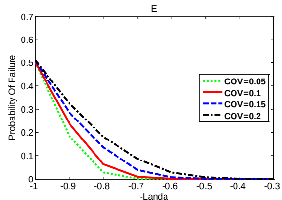
شکل ۹- محاسبه احتمال خرابی در سطوح مختلف نیرو کم‌انرژی و تأثیر پارامتر E (برای شکل (۸))
