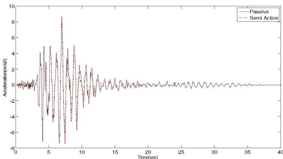
شکل ۴- نمودار تاریخچه زمانی پاسخ شتاب سازه تحت اثر زلزله حوزه نزدیک نرتریج
