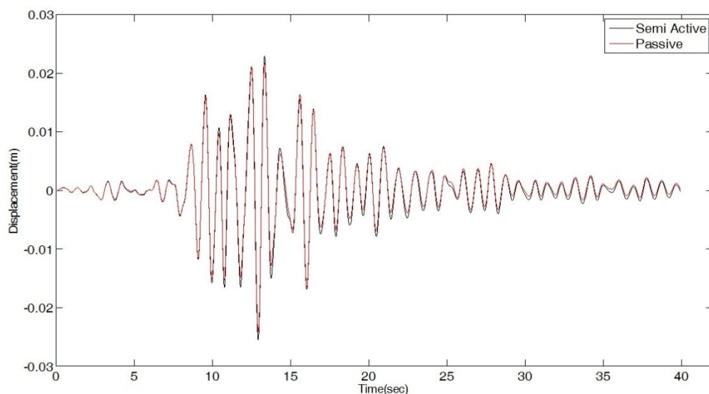
شکل ۶- نمودار تاریخچه زمانی پاسخ جابجایی سازه تحت اثر زلزله حوزه دور لوماپریتا (کلیف هوس)
