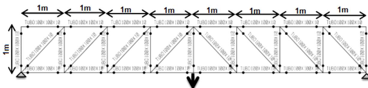
شکل ۶- نمایی از خرابای دو بعدی، مقاطع اعضا و ابعاد
