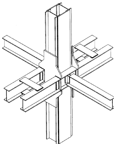
شکل ۲- اتصال فولادی پیشنهادی توسط Faridmehr و همکارانش [۱۴]
