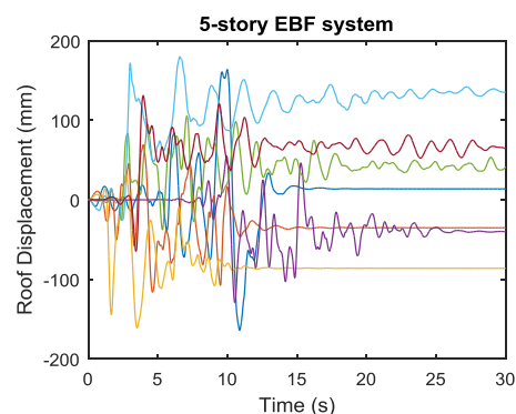
الف) سازه ۵ طبقه متداول
