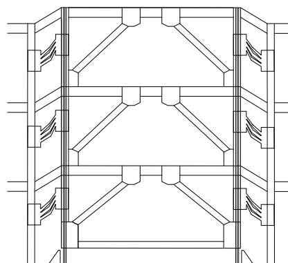
شکل ۳- بلندشدگی کامل قاب
