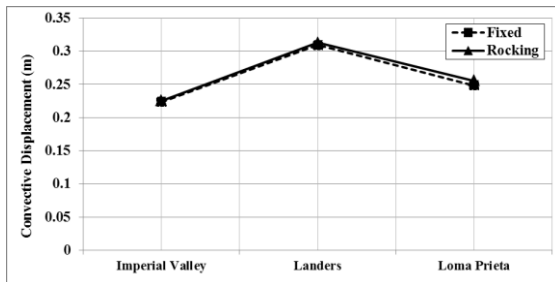
شکل ۷- مقایسه بیشینه تغییر مکان جرم نوسانی مخزن مهار شده و مخزن با رفتار گهواره‌ای تحت اثر شتاب‌نگاشت‌های مختلف
