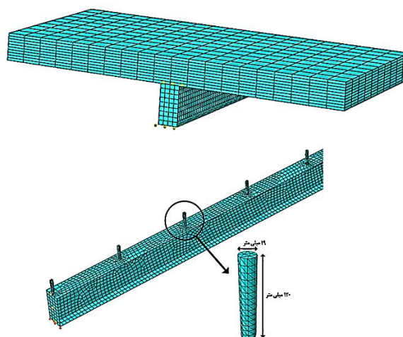
شکل ۲- شکل هندسی تیر و دال مختلط به همراه برشگیر
