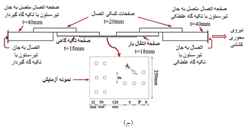
شکل ۳- جزئیات نحوه آزمایش، (الف) ستاپ آزمایش (Test set-up)، (ب) جزئیات نصب LVDTها روی نمونه آزمایش، و (ج) شماتیک نحوه اعمال بار و جزئیات هندسی نمونه‌ها
