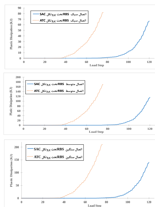
شکل ۱۴- مقایسه انرژی پلاستیک مستهلک شده در تمام تیپ‌های اتصالات سازه ۷ طبقه تحت پروتکل بارگذاری SAC و ATC-24 در تغییر مکان پذیرش
