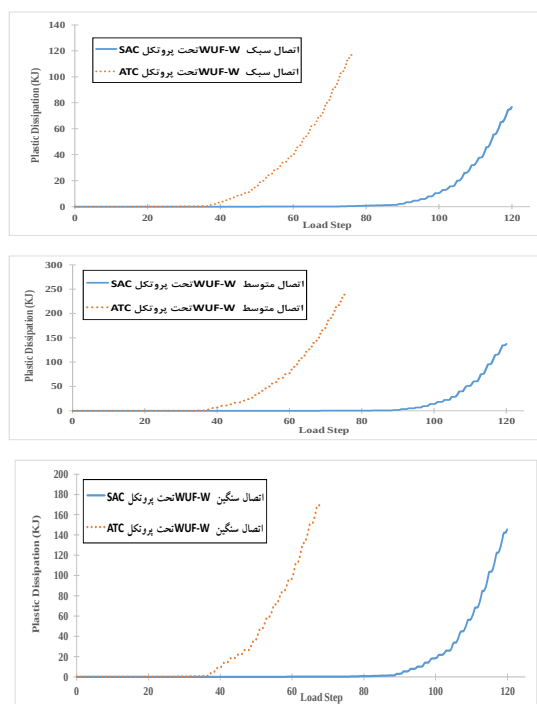
شکل ۱۴- مقایسه انرژی پلاستیک مستهلک شده در تمام تیپ‌های اتصالات سازه ۷ طبقه تحت پروتکل بارگذاری SAC و ATC-24 در تغییر مکان پذیرش
