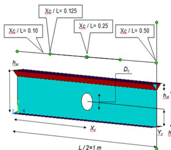
شکل ۳- موقعیت مکانی پارامترهای تعریف شده برای نصف طول تیورق (تیورق مقارن می‌باشد).
