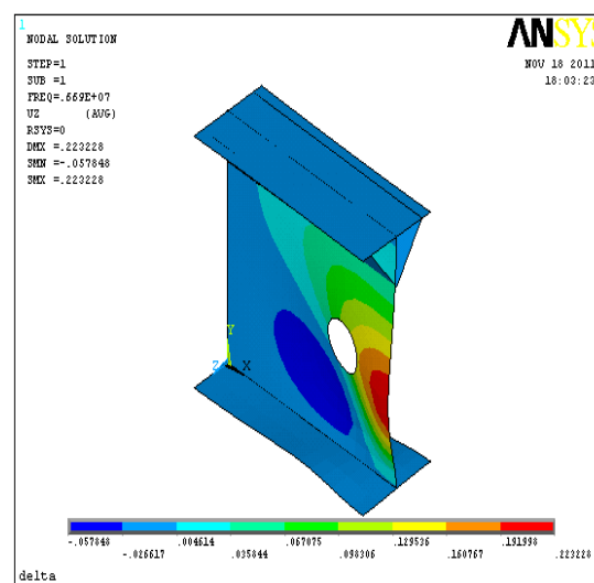
شکل ۷- توزیع تنش به صورت قطری در جان تیرورق ( X_c/L = 0/3 )
