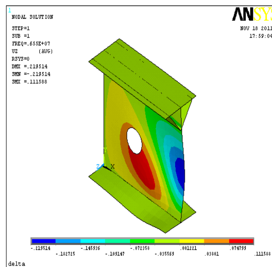
شکل ۶- توزیع تنش به صورت قطری در جان تیرورق ( X_c/L = 0/2 )
