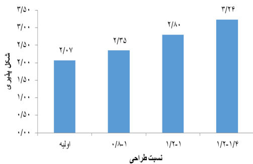
شکل ۱۳- مقایسه شکل پذیری در حالت های مختلف طراحی برای قاب ۲ دهانه ۲ طبقه با المان خمشی
