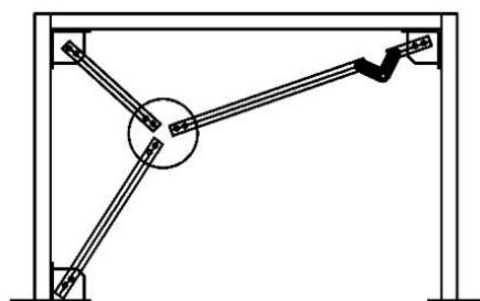
(ب) قاب ۷ شکل با میراگر اصطکاکی دورانی نوع دوم
