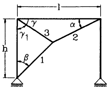
شکل ۳- مهاربند برون محور [۸]
