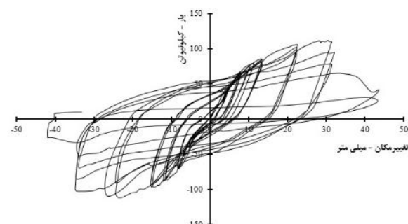
ج) CFST-D
