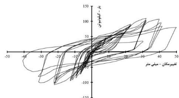
ب) CFST-S
