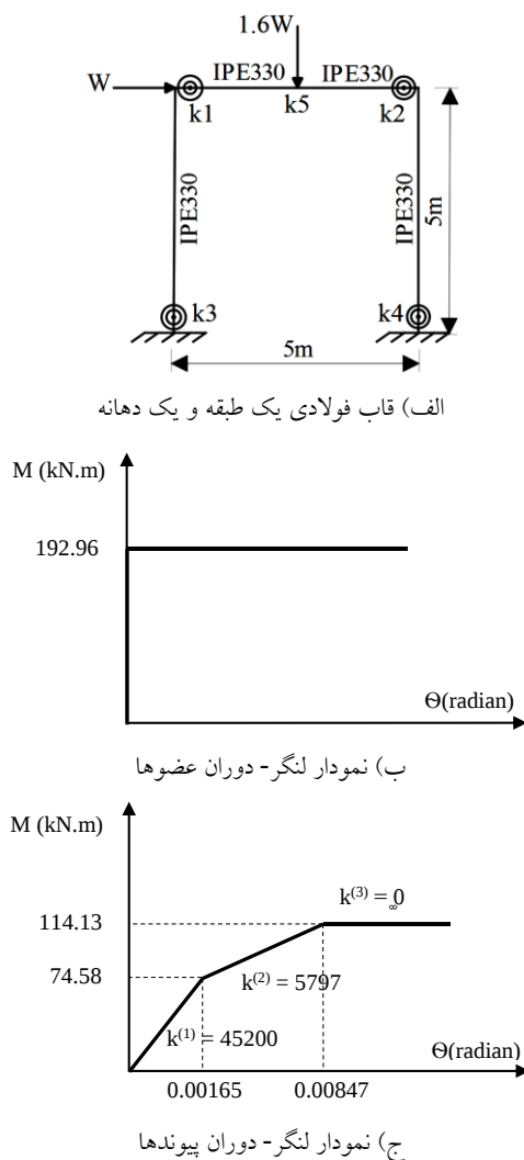
شکل ۱- قاب فولادی یک طبقه و یک دهانه و رفتار کشسان-مومسان اعضا و پیوندها [۱۸]
