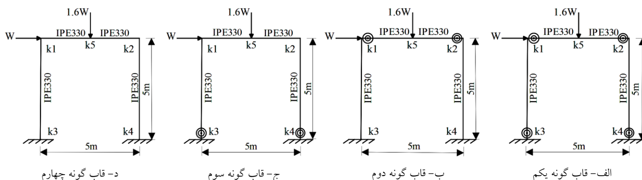
شکل ۲- قاب یک طبقه- یک دهانه ( F1 ) با پیوندهای متفاوت عضو و تکیه‌گاهی
