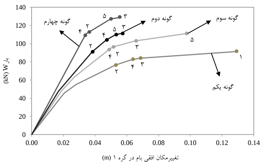
شکل ۴- نمودار بار- تغییر مکان و ترتیب شکل‌گیری مفصل‌های خمیری در گونه‌های متفاوت قاب یک طبقه- یک دهانه (F1)
