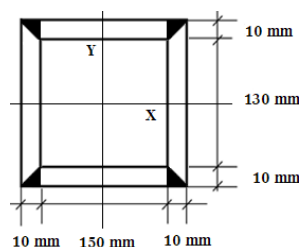
شکل ۳- مقطع ستون ساخته شده با جوش گوشه در اتصال کنج برای نمونه مورد آزمایش
