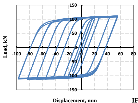
شکل ۱۳- منحنی نیرو-جابجایی (هیسترزیس) برای نمونه قاب خمشی متوسط با ستون جعبه‌ای ساخته شده با جوش گوشه (IF)
