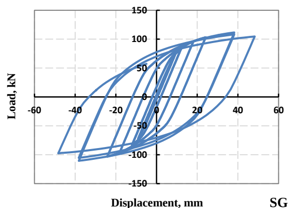
شکل ۱۰- منحنی نیرو-جابجایی (هیسترزیس) برای نمونه قاب خمشی ویژه با ستون جعبه‌ای ساخته شده با جوش شیاری (SG)
