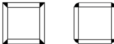
(ب) جوش شیار با نفوذ کامل
