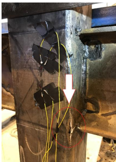
شکل ۸- نمونه قاب خمشی متوسط با جوش گوشه (IF) و گسیختگی جوش ستون ناحیه چشمه اتصال پس از اعمال بارگذاری در جابجایی نسبی ۹۶ میلی متر
