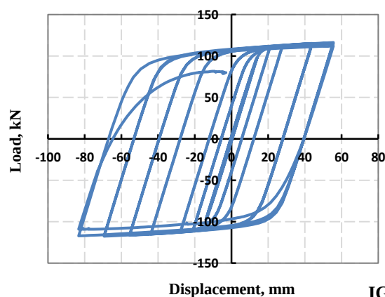
شکل ۱۲- منحنی نیرو-جابجایی (هیسترزیس) برای نمونه قاب خمشی متوسط با ستون جعبه‌ای ساخته شده با جوش شیاری (IG)
