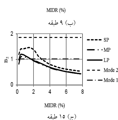
شکل ۶- تغییرات متغیر B_2 برحسب MIDR برای قاب‌های مورد مطالعه
