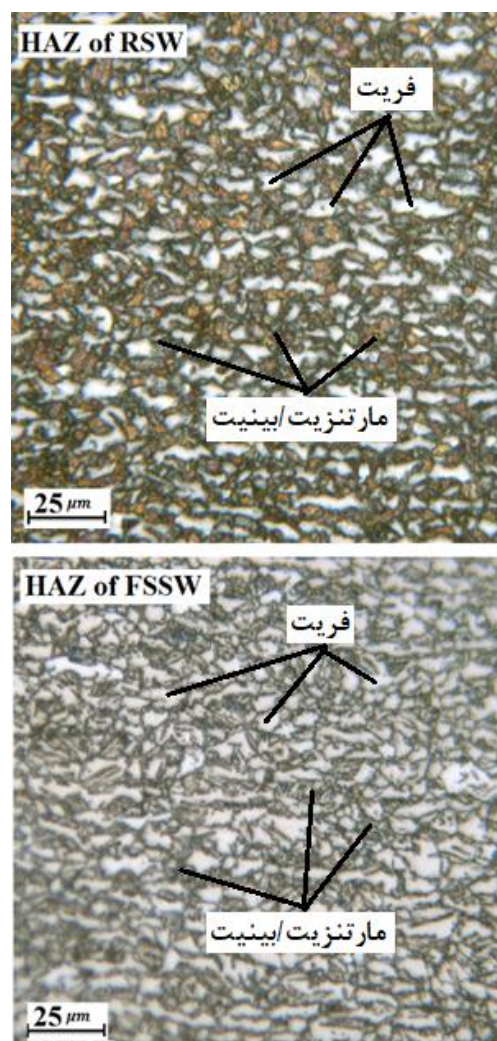
شکل ۹- ریزساختار میکروسکوپ نوری ناحیه HAZ برای دو روش (نواحی روشن فاز فریت و نواحی تیره فاز مارتنزیت/بینیت می‌باشند).
