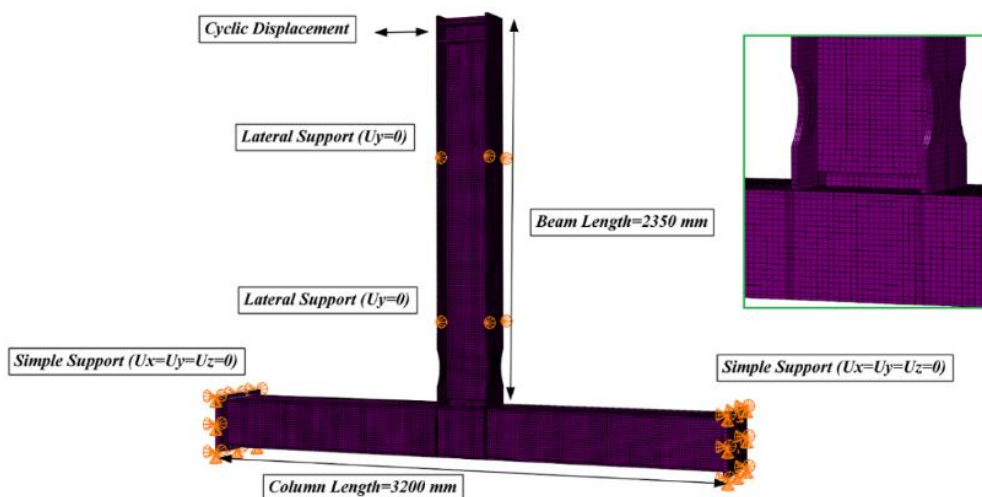
شکل ۲۵- مدل عددی تپ آزمایشگاهی اتصال RBS در نرم افزار ABAQUS
