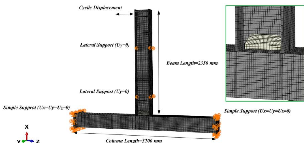
شکل ۲۴- مدل عددی تپ آزمایشگاهی اتصال WUF-W در نرم افزار ABAQUS
