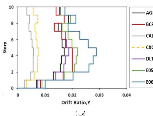
شکل ۶- پوش بیشینه جابجایی نسبی طبقات در راستای Y پلان: (الف) سازه Bundled Tube و (ب) سازه 3D FRAME (شکل (۳))
