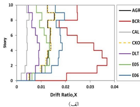
شکل ۵- پوش بیشینه جابجایی نسبی طبقات در راستای X پلان: (الف) سازه Bundled Tube و (ب) سازه 3D FRAME (شکل (۳))
