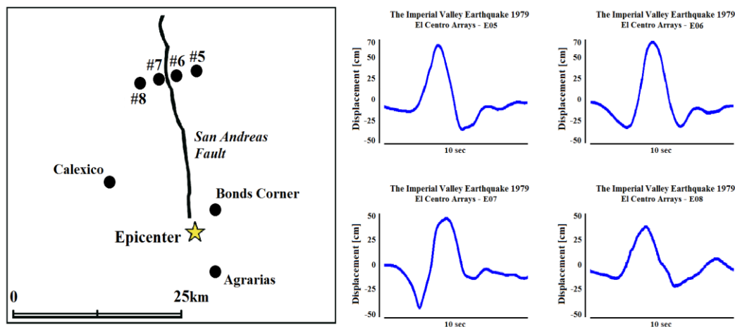
شکل ۱- حوزه لرزه خیز دره امپریال در زلزله ۱۹۷۹ کالیفرنیا و نمایش پالس‌های برداشته و پیوسته تغییر مکان متناظر با مولفه TR رکورد ایستگاه‌های E05، E06، E07 و E08
