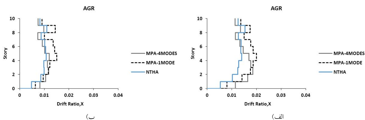
شکل ۹- پوش بیشینه دررفت در راستای X تحت رکورد مقیاس شده AGR: (الف) سازه Bundled Tube و (ب) سازه 3D FRAME (شکل ۳)
