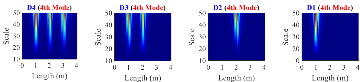
شکل ۷- نمودار دو بعدی ضرایب موجک سیگنال ورودی مود چهارم حالت‌های آسیب D1 تا D4
