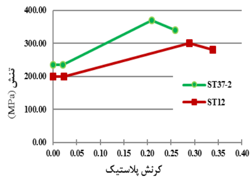
شکل ۹- نمودار تنش-کرنش پلاستیک مصالح ST12 و ST37
