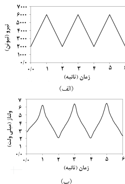
شکل ۱۱- پاسخ حسگر به بار مثلثی تناوبی با دامنه‌ی تغییرات ۴۰۰۰ نیوتن و زمان تناوب ۲ ثانیه: (الف) نیرو- زمان و (ب) ولتاژ- زمان
