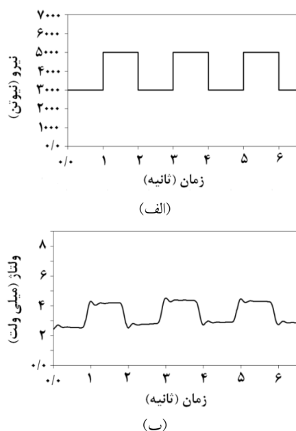
شکل ۱۲- پاسخ حسگر به بار مستطیلی تناوبی با دامنه‌ی تغییرات ۲۰۰۰ نیوتن و زمان تناوب ۲ ثانیه: (الف) نیرو- زمان و (ب) ولتاژ- زمان
