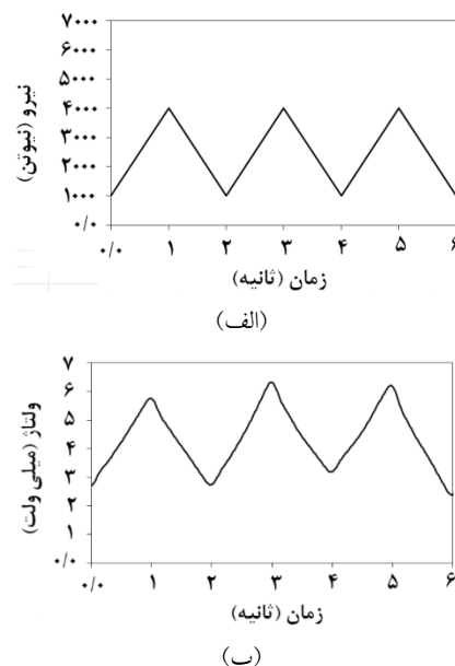
شکل ۱۰- پاسخ حسگر به بار مثلثی تناوبی با دامنه‌ی تغییرات ۳۰۰۰ نیوتن و زمان تناوب ۲ ثانیه: (الف) نیرو- زمان، (ب) ولتاژ- زمان
