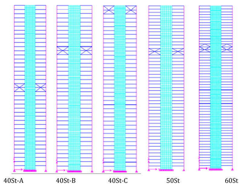
شکل ۳- موقعیت قرارگیری مهار بازویی در مدل طراحی
