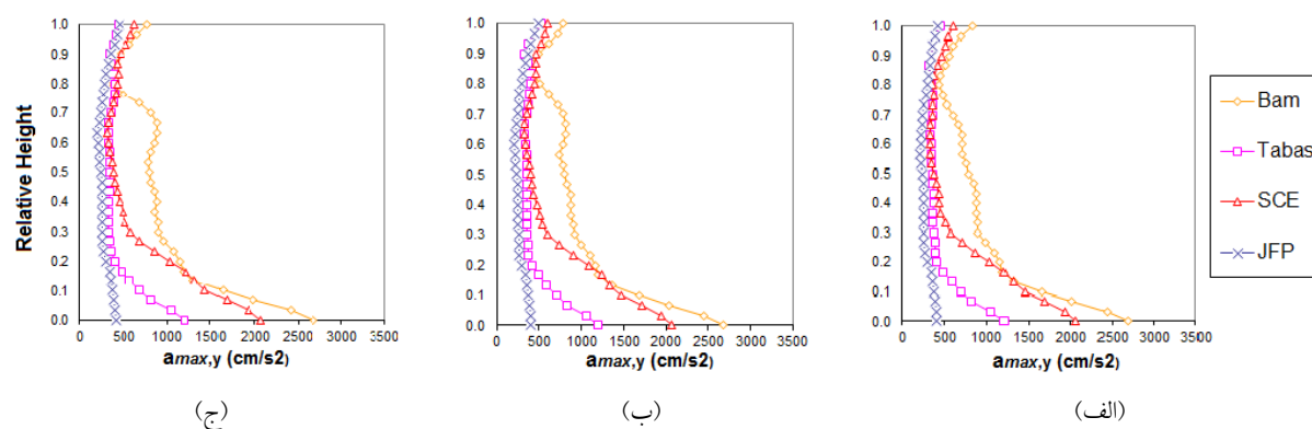
شکل ۹- پوش ماکزیمم شتاب مطلق طبقات در سازه‌های مطالعاتی ۳۰ طبقه: (الف) مدولاسیون یکنواخت، (ب) مدولاسیون ۵ طبقه‌ای و (ج) مدولاسیون ۴ طبقه‌ای
