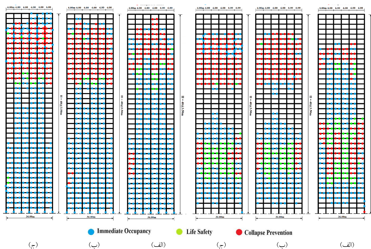
شکل ۲۱- ساختار مفصل پلاستیک در سازه‌های مطالعاتی ۴۰ طبقه در انتهای بازه زمانی رکورد SCE: (الف) مدولاسیون یکنواخت، (ب) مدولاسیون ۵ طبقه‌ای و (ج) مدولاسیون ۴ طبقه‌ای (تعریف سطوح عملکرد بر اساس Fema 356 می‌باشد.)
