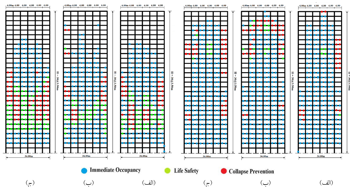
شکل ۱۹- ساختار مفصل پلاستیک در سازه‌های مطالعاتی ۳۰ طبقه در انتهای بازه زمانی رکورد SCE: (الف) مدولاسیون یکنواخت، (ب) مدولاسیون ۵ طبقه‌ای و (ج) مدولاسیون ۴ طبقه‌ای (تعریف سطوح عملکرد بر اساس Fema 356 می‌باشد).
