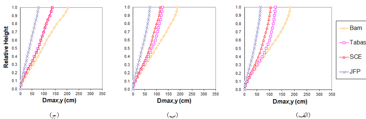
شکل ۱۱- پوش ماکزیمم تغییرمکان طبقات در سازه‌های مطالعاتی ۲۰ طبقه: (الف) مدولاسیون یکنواخت، (ب) مدولاسیون ۵ طبقه‌ای و (ج) مدولاسیون ۴ طبقه‌ای
