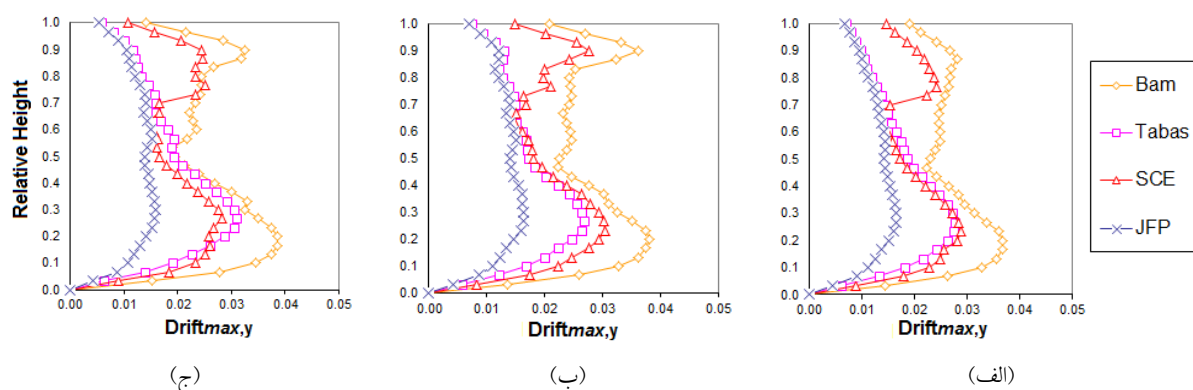
شکل ۱۵- پوش ماکزیمم دریفت طبقات در سازه‌های مطالعاتی ۳۰ طبقه: (الف) مدولاسیون یکنواخت، (ب) مدولاسیون ۵ طبقه‌ای و (ج) مدولاسیون ۴ طبقه‌ای
