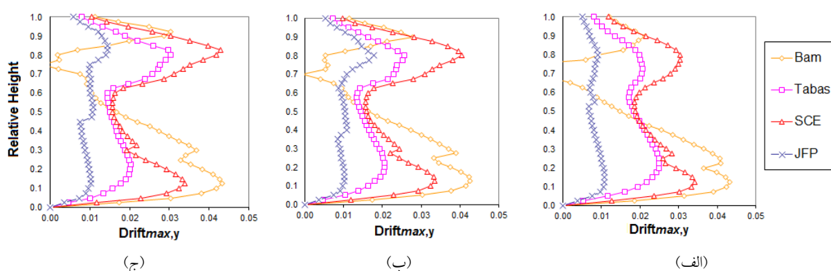
شکل ۱۶- پوش ماکزیمم دریفت طبقات در سازه‌های مطالعاتی ۴۰ طبقه: (الف) مدولاسیون یکنواخت، (ب) مدولاسیون ۵ طبقه‌ای و (ج) مدولاسیون ۴ طبقه‌ای
