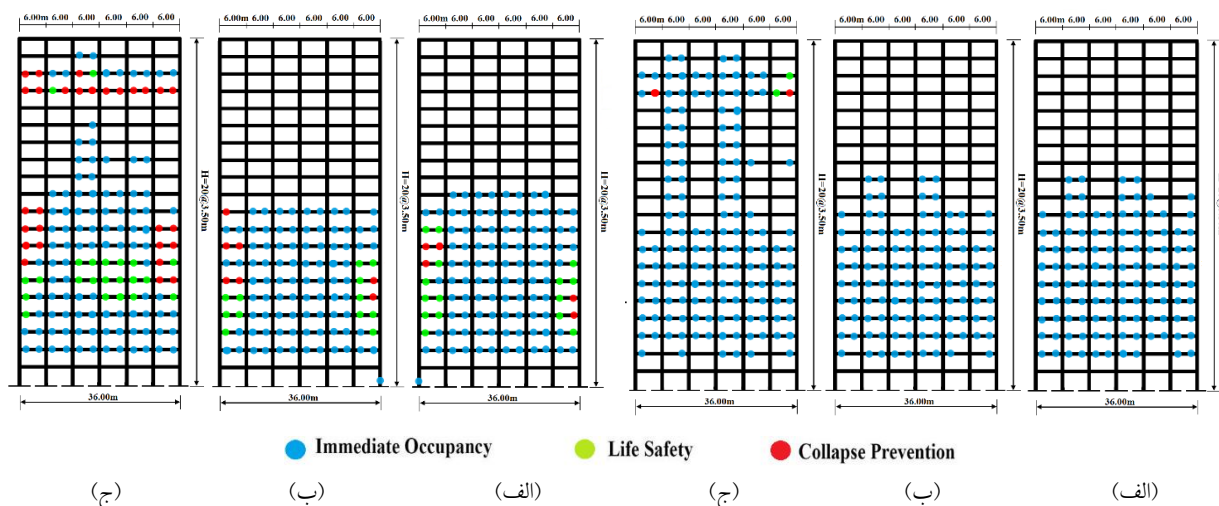
شکل ۱۷- ساختار مفصل پلاستیک در سازه‌های مطالعاتی ۲۰ طبقه در انتهای بازه زمانی رکورد SCE: (الف) مدولاسیون یکنواخت، (ب) مدولاسیون ۵ طبقه‌ای و (ج) مدولاسیون ۴ طبقه‌ای (تعریف سطوح عملکرد بر اساس Fema 356 می‌باشد).
