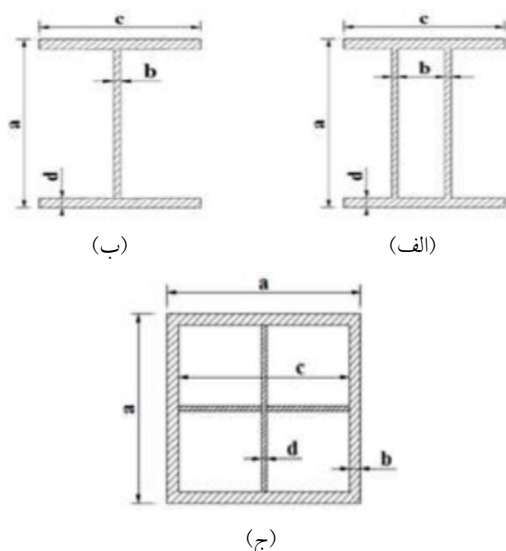
شکل ۲- مقاطع المان‌های سازه‌های مطالعاتی؛ (الف) نیمرخ المان‌های تیر در سازه‌های مطالعاتی ۳۰ و ۴۰ طبقه B \times b \times c \times d ، (ب) نیمرخ المان‌های تیر در سازه‌های مطالعاتی ۲۰ طبقه B \times b \times c \times d ، (ج) نیمرخ ستون‌ها همراه با بخش سخت کننده داخلی در پنج طبقه اول سازه‌های ۳۰ و ۴۰ طبقه C \times a \times b \times c \times d [۴۰]
