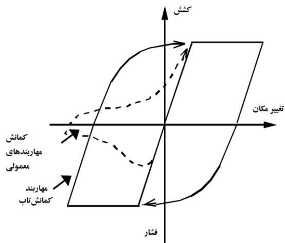
شکل (۱): رفتار کشش و فشار محوری مهاربند کمناش تاب
