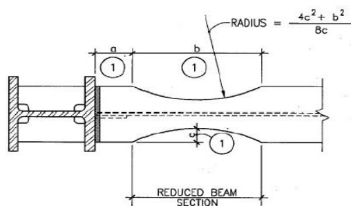
شکل ۴- هندسه‌ی تیر با مقطع کاهش یافته [۲۳]
