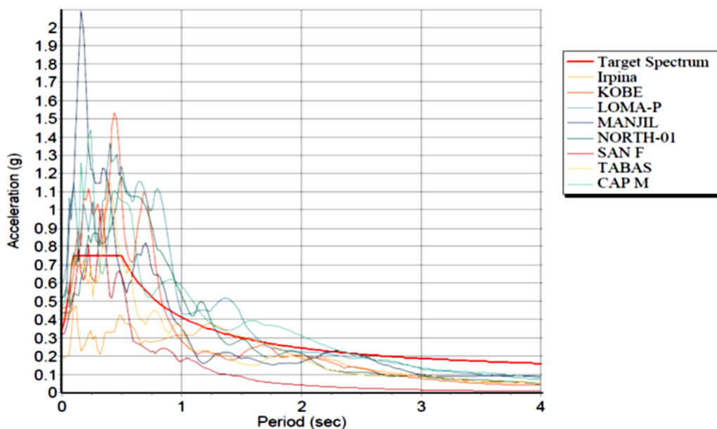
شکل ۷- نمودار رکورد زلزله‌های انتخابی مقیاس‌نشده و طیف طرح استاندارد ۲۸۰۰
