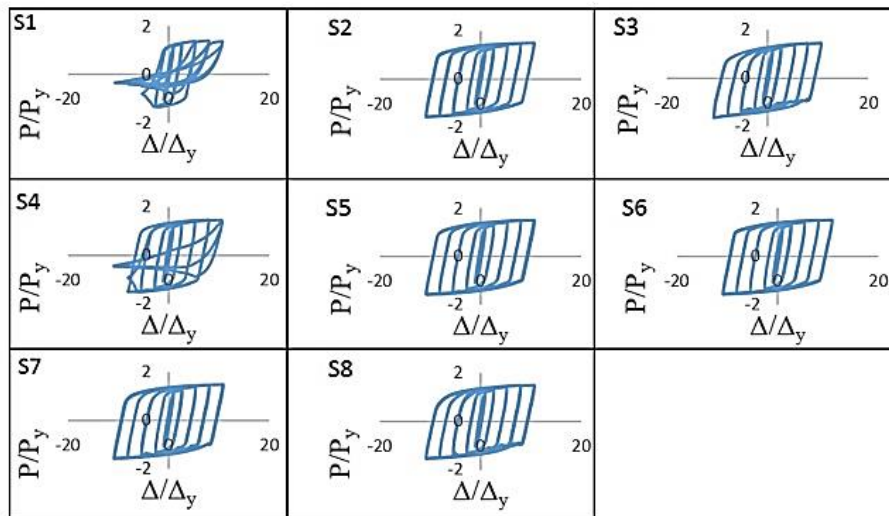
شکل ۱۰- منحنی های هیستریزیس به دست آمده از نمونه ها
