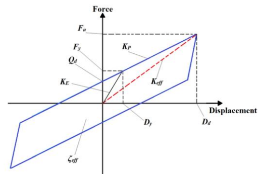
شکل ۳- شماتیک حلقه هیسترتیک (رفتار نیرو-تغییر شکل دوخطی جداگر LRB)
