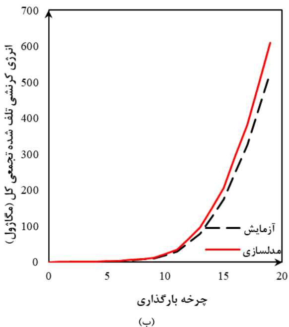
شکل ۶- مقایسه (الف) نمودار هیستریزیس و (ب) اتلاف انرژی کرنشی تجمعی کل نمونه مدل‌شده در مقاله حاضر با نمونه آزمایشگاهی مربوط به مرجع [۳]
