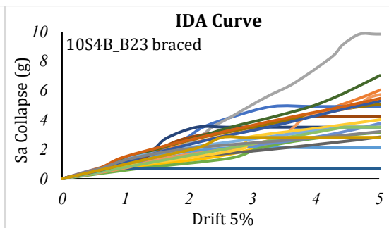
شکل ۱۷- نمودار تحلیل دینامیکی افزایشی قاب چهار دهانه با دهانه‌های ۲ و ۳ مهاربندی
