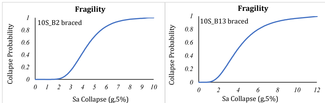
شکل ۱۲- منحنی شکنندگی قاب سه دهانه با دهانه وسط
