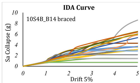
شکل ۱۸- نمودار تحلیل دینامیکی افزایشی قاب چهار دهانه با دهانه‌های ۱ و ۴ مهاربندی
