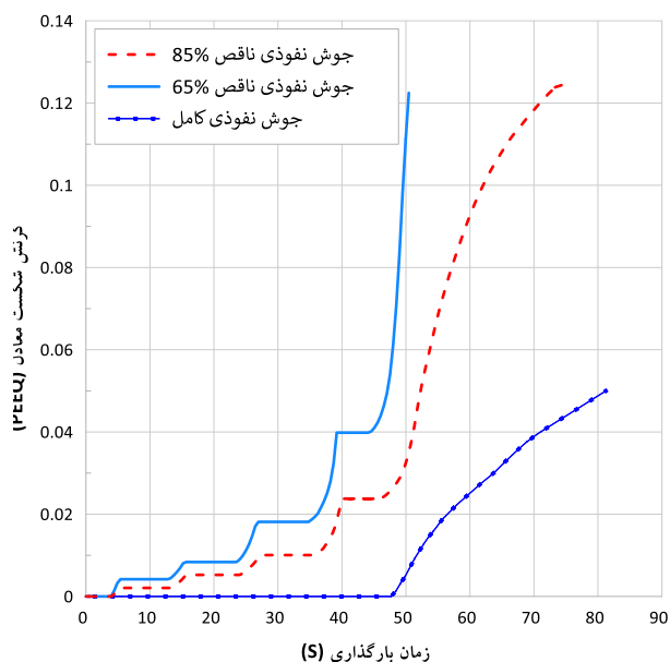
الف) وصله ستون قوطی شکل با پهنای ۳۰۰ میلی متر دارای دو ضخامت مختلف ۲۵ و ۳۰ میلی متر
