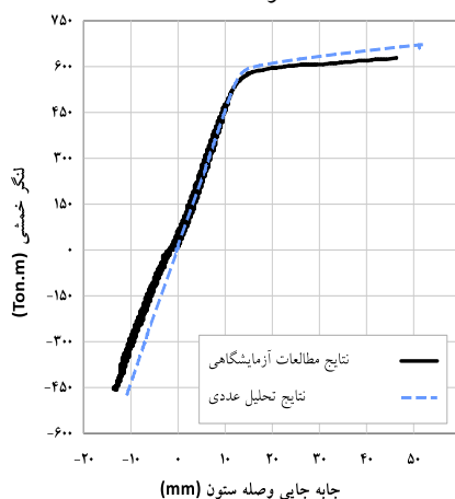
شکل ۱۰- مقایسه منحنی لنگر خمشی-جابه‌جایی محل وصله ستون در نمونه‌های مدل‌سازی‌شده و نمونه‌های آزمایشگاهی شاور و کانوینده
