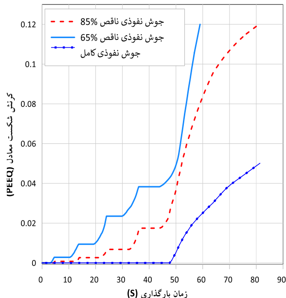
ب) وصله ستون قوطی شکل با پهنای ۳۰۰ میلی متر دارای دو ضخامت یکسان ۳۰ میلی متر
