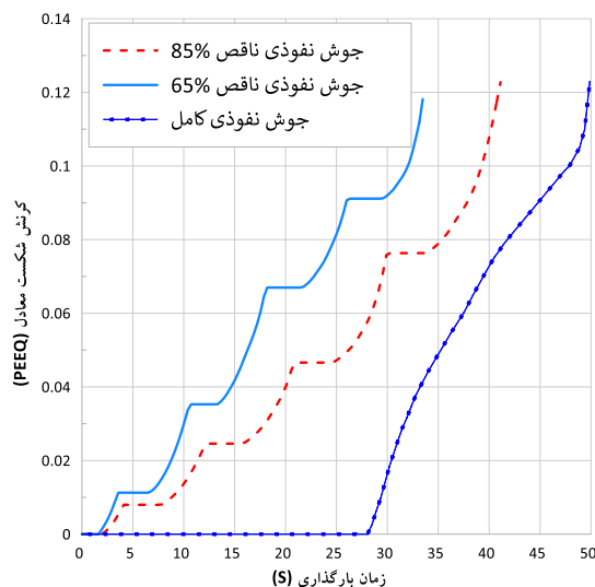
شکل ۱۵- تغییرات کرنش شکست معادل در المان بحرانی (پ) وصله ستون قوطی شکل با پهنای ۵۰۰ میلی متر دارای دو ضخامت مختلف ۳۰ و ۴۰ میلی متر
