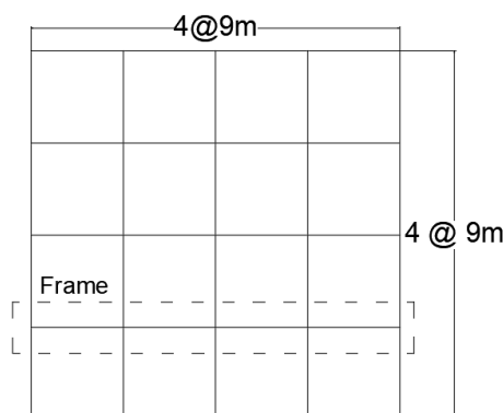
شکل ۴- پلان طبقات ساختمان و موقعیت قرارگیری قاب خمشی مورد بحث
