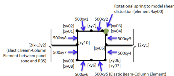
شکل ۲- مدل مفهومی چشمه‌های اتصال قاب خمشی
