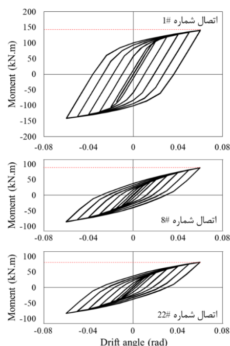
شکل ۱۹- منحنی های رفتار چرخه ای اتصالاتی دارای یک میراگر و اتصال دارای دو میراگر با قطر پیچ تسلیمی ۱۸/۵ میلی متر
