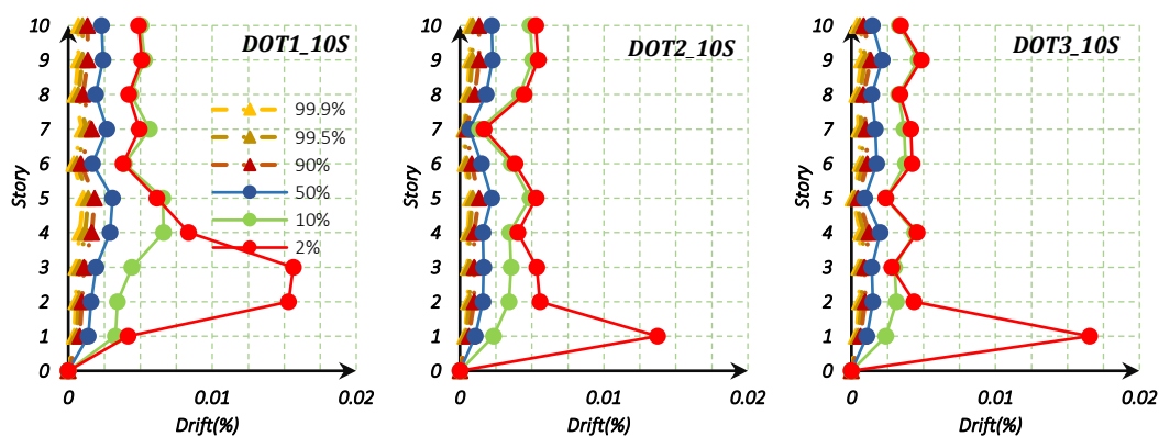
شکل ۶- نمودار جابه‌جایی نسبی طبقات برای قاب‌های DOT1، DOT2 و DOT3 بهینه‌سازی شده بر اساس عملکرد با دهانه‌های کناری مهاربندی
