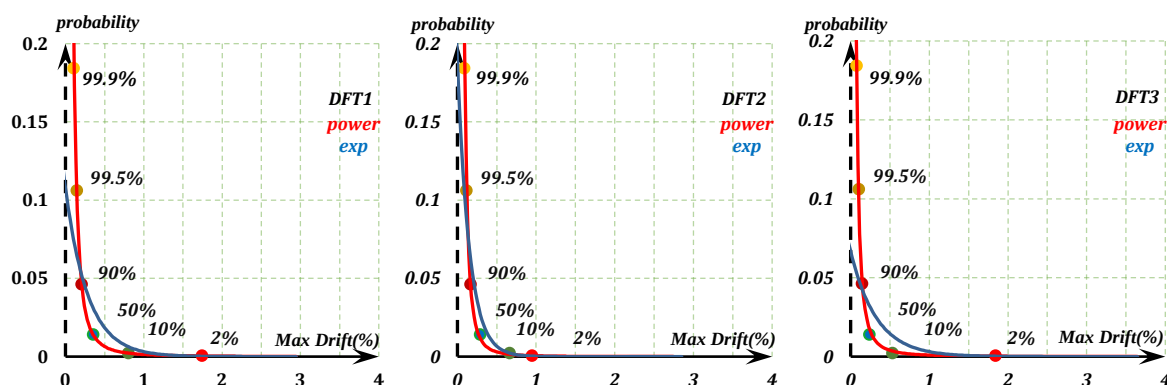
شکل ۷- نمودار برازش منحنی احتمال وقوع در برابر دررفت متناظر برای قاب‌های DFT1، DFT2 و DFT3 بهینه‌سازی شده بر اساس عملکرد با دهانه وسط مهاربندی در سطوح عملکردی متناظر سطوح خطر ۹۹/۹، ۹۹/۵، ۹۰، ۵۰، ۲٪ و ۵۰ سال
