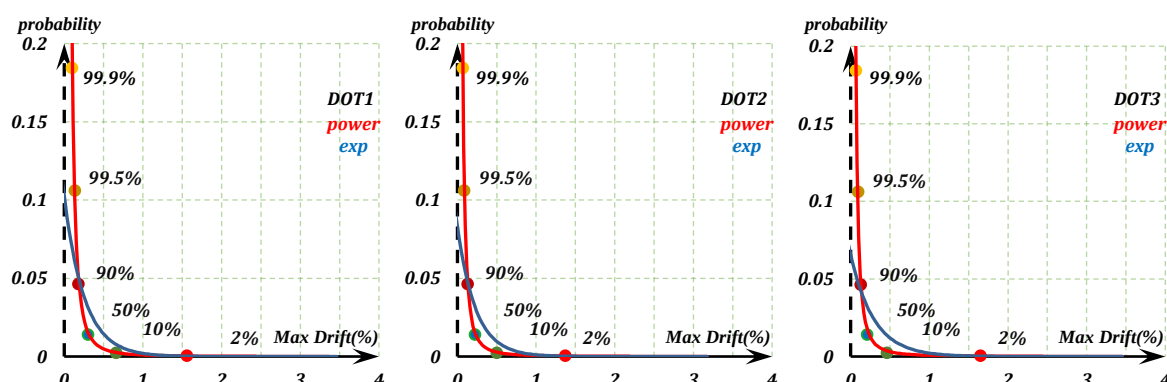
شکل ۸- نمودار برازش منحنی احتمال وقوع در برابر دررفت متناظر برای قاب‌های DOT1، DOT2 و DOT3 بهینه‌سازی شده بر اساس عملکرد با دهانه کناری مهاربندی در سطوح عملکردی متناظر سطوح خطر ۹۹/۹، ۹۹/۵، ۹۰، ۵۰، ۲٪ و ۵۰ سال
