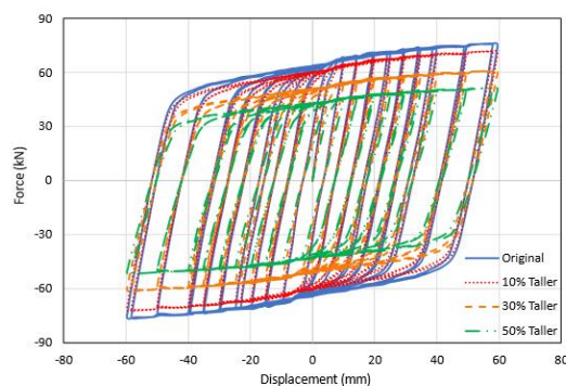
شکل ۱۸- اثر افزایش ارتفاع میراگر بر منحنی هیستریزیس
