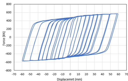
شکل ۳۳- منحنی هیستریزیس دو میراگر بر روی هم
