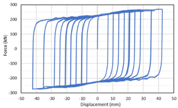
شکل ۳۰- منحنی هیستریزیس میراگر در جهت عمود بر حرکت
