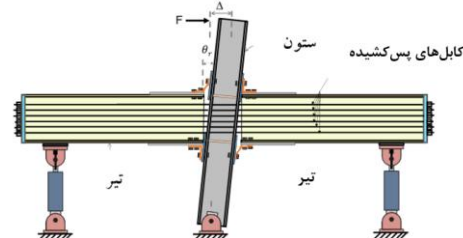
شکل ۶- شماتیک نمونه مدل سازی شده
