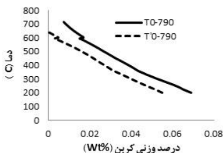
شکل (۷): نمودارهای T'0 و T_0 برای T_{IA}=790^\circ\text{C}
