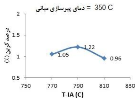
شکل (۶): در صد وزنی کربن در آستنیت باقیمانده در
