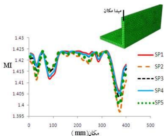
شکل ۱۷- تغییرات شاخص میسر در طول ناحیه بحرانی شماره (۲) نبشی کششی پنج مدل اتصال پس کشیده
