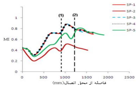
شکل ۱۳- چگونگی تغییرات شاخص میسر در طول خط مرکزی بال تیر پنج مدل مورد بررسی
