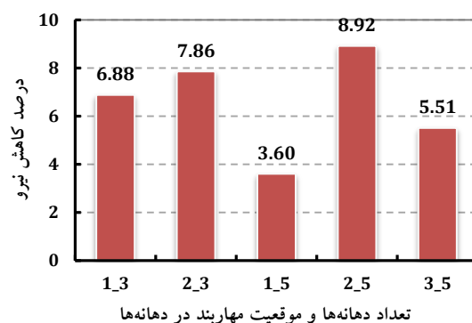
شکل ۷- درصد کاهش برش پایه در قاب‌های سه طبقه با سه و پنج دهانه با مهارند قطری با مقطع کاهش یافته به نسبت قاب با مهارند قطری معمولی در دهانه‌های مختلف
