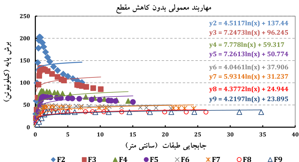
شکل ۹- منحنی بار-جابجایی قاب‌های دو تا نه طبقه در حالت قاب با مهارند بدون کاهش مقطع (کیلونوتن-سانتی متر)
