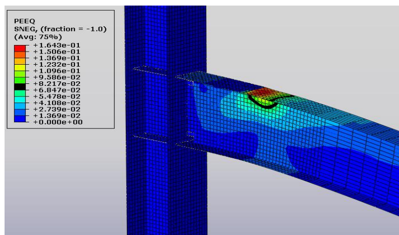
شکل (۱۱): کانتور کرنش پلاستیک مدل تقویت شده برای صحت سنجی
