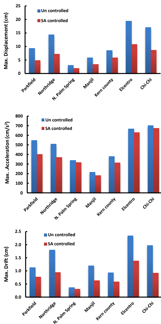
شکل ۱۱- نمودار مقادیر کاهش در پاسخهای سازه دوازده طبقه
