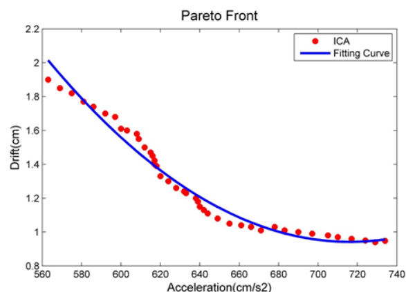
شکل ۸- جبهه بهینه پارتو برای حداکثر شتاب طبقات و حداکثر جابه‌جایی نسبی طبقات
