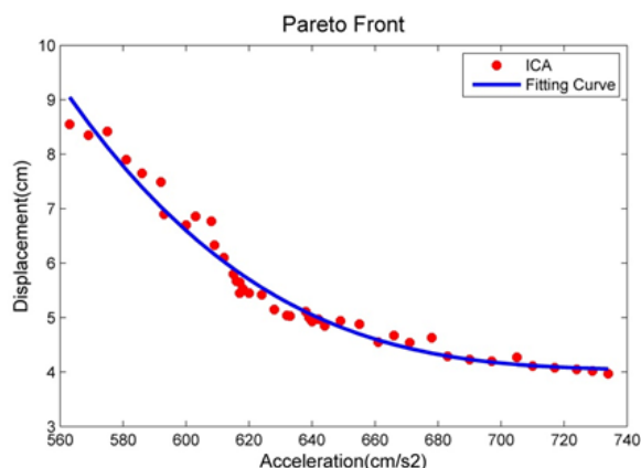
شکل ۷- جبهه بهینه پارتو برای حداکثر شتاب طبقات و حداکثر جابه‌جایی طبقه آخر
