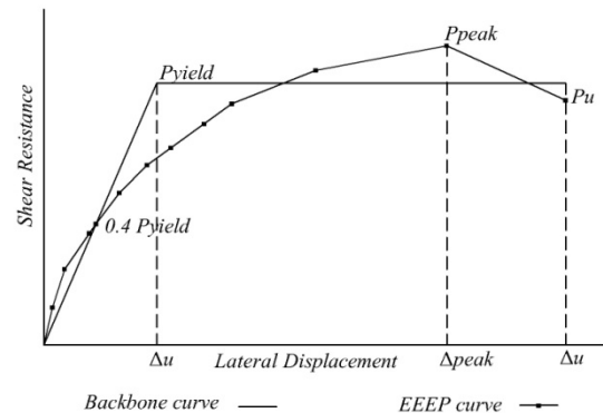
شکل (۱۱): محاسبه تغییر مکان جانبی نهایی و حد تسلیم منحنی پوش بار-تغییر مکان جانبی بر اساس استاندارد ASTM E2126-07
