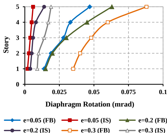
شکل ۱۲- میانگین بیشینه دوران طبقات برحسب مقادارهای مختلف برون محوری سختی
