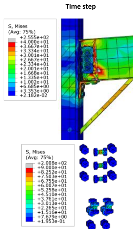
شکل ۱۵- نمودار تغییر مکان-زمان مدل پنج، منحنی تنش و تغییر شکل نهایی اتصال
