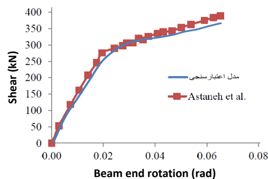
شکل ۹- مقایسه ای از منحنی برش-دوران تیر نمونه آزمایشگاهی انجام شده توسط Astaneh و همکارانش [۲۰] و مدل اعتبارسنجی
