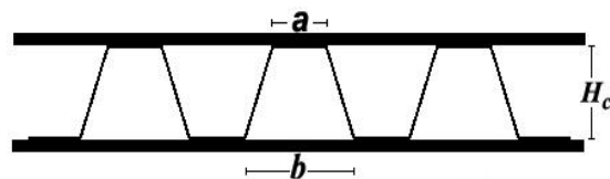
شکل ۲- شکل هندسی پانل کنگره‌ای مورد استفاده برای صحت‌سنجی و پارامترهای هندسی آن
