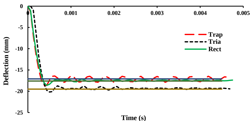
شکل ۱۳- تغییر شکل مرکز ورق پشتی پانل، در پانل‌های تمام آلومینیومی
