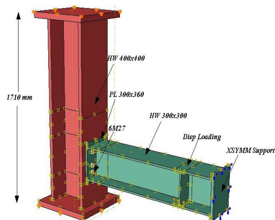
شکل ۸- نمونه مدل عددی ساخته شده براساس [۲۹]
