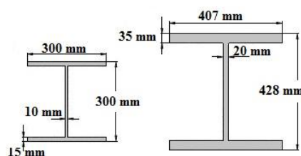
شکل ۶- جزئیات مقطع ستون و تیر [۳۲]
