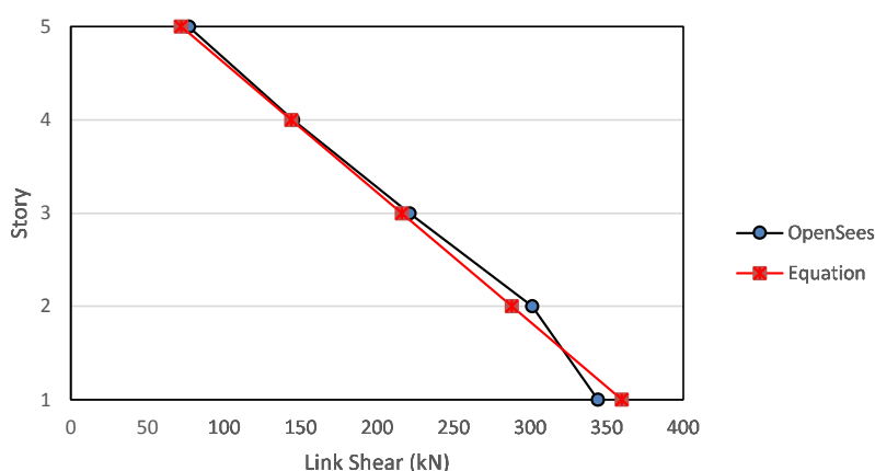
شکل ۷- برش تیرپیوند در هر طبقه
